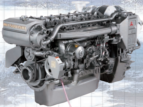
IMO Tier 2 NOx規制適合 S6M3F-T2MTKL MAX.279kW(380PS)
